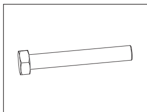
26 - BULLONE M10x70 - 8pz
