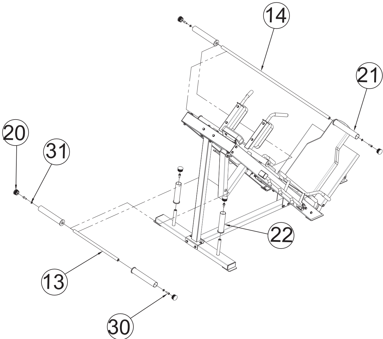
22 - PORTA DISCHI PESO - 2pz
