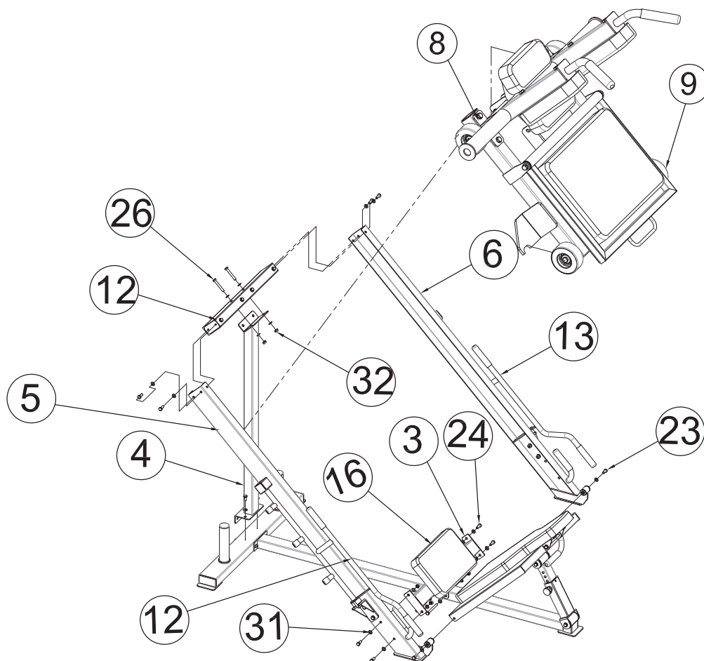
31 - RONDELLA - 18pz
