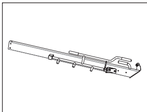
5 - TELAIO DESTRO - 1pz
